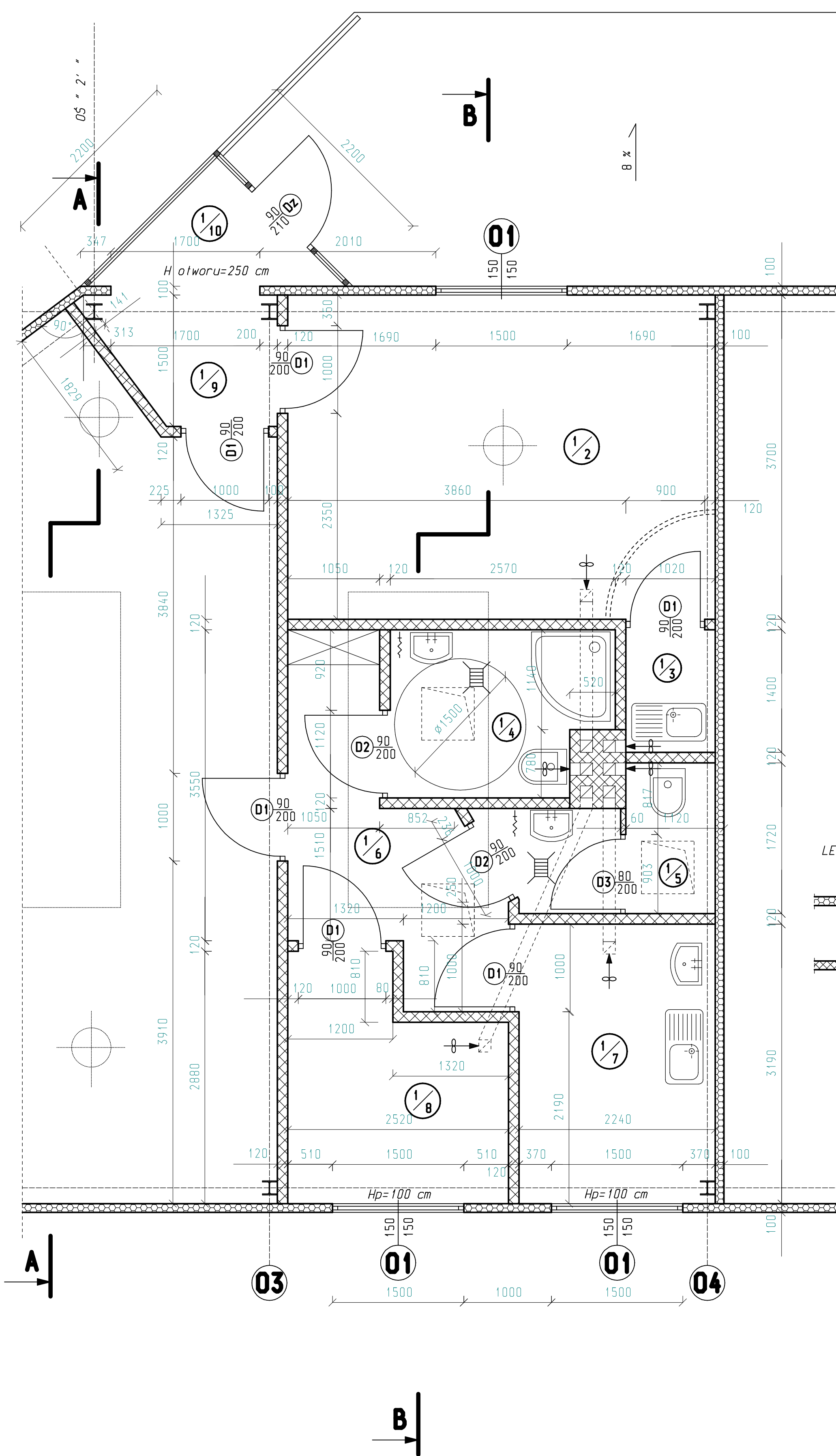
RZUT ZAPLECZA BIUROWO-SOCJALNEGO SEGMENTU 1 skala 1:50
